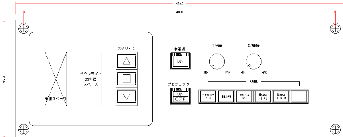
操作パネル
